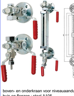
fig 892 plexiglas lengte 1 m diam. 10 - 13 - 16 - 18 - 20 mm fig 893 pyrex glas lengte 1,5 m diam. 10 - 13 - 14 - 16 - 18 - 20 mm fig 894 messing beschermhuis U lengte 1 m diam. 10 - 13 - 16 - 18 - 20 mm temp. : max +80°C
